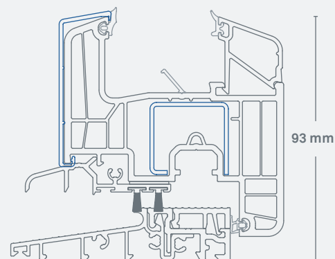
Novinka: Bezbariérový práh balkonových dveří / Obr.: 1:2
