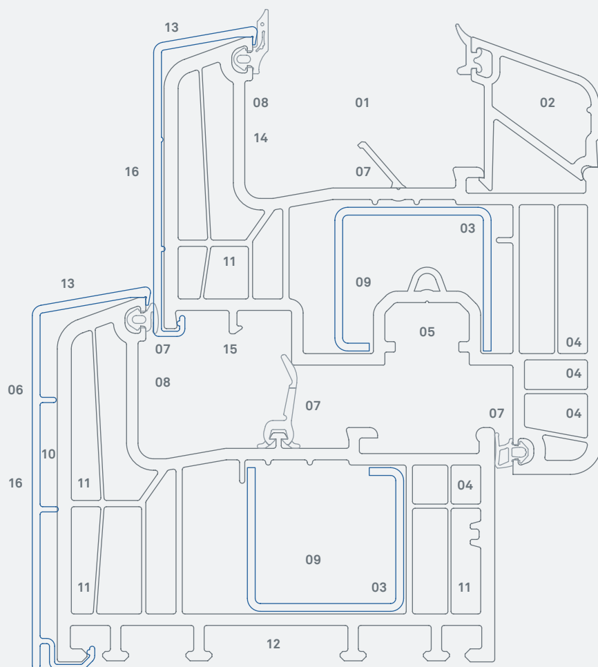
Eforte s hliníkovým krytem Obr.: 1:1
